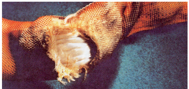
Bild 4-6: Beschädigung durch Hitze einwirkung; Ablegereife auch wegen Sichtbarkeit der Einlage erreicht
