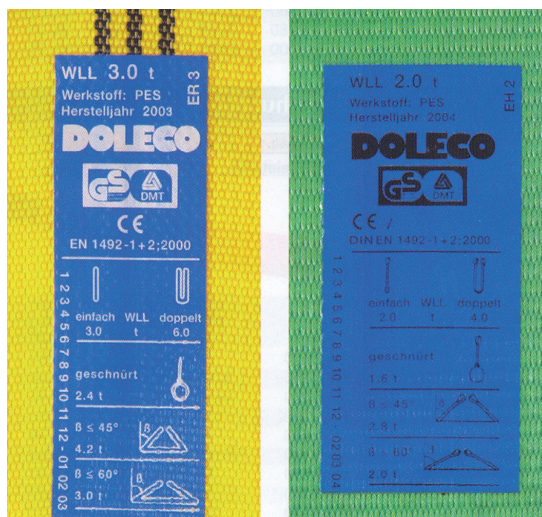
Bild 1-2: Angaben auf Etikett beachten
