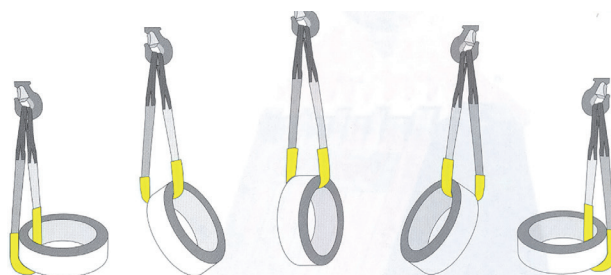
Bild 1-7: Wenden von Coils
