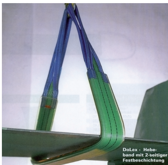
Bild 1-6: Kantenschutz - Festbeschichtung
