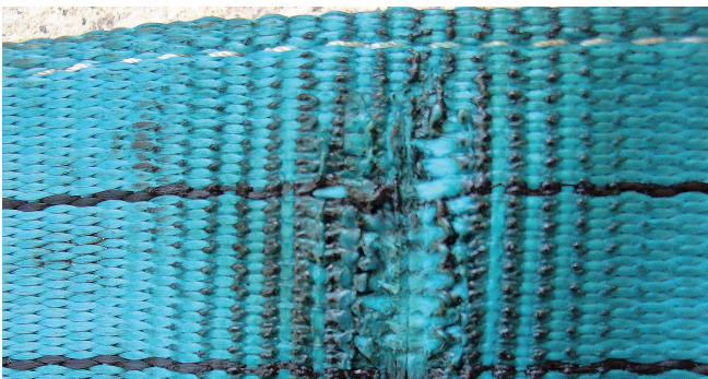
Bild 4-3: Durch Wärmeeinfluss beschädigte Oberfläche
